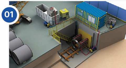
추진 기지 및 플랜트 설치
