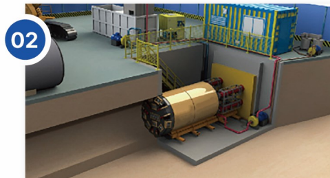
Micro TBM 장비설치
