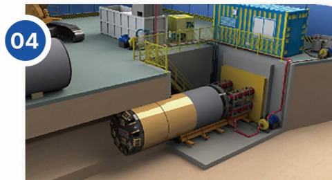
추진장비 굴진 및 후방 배관 연결
